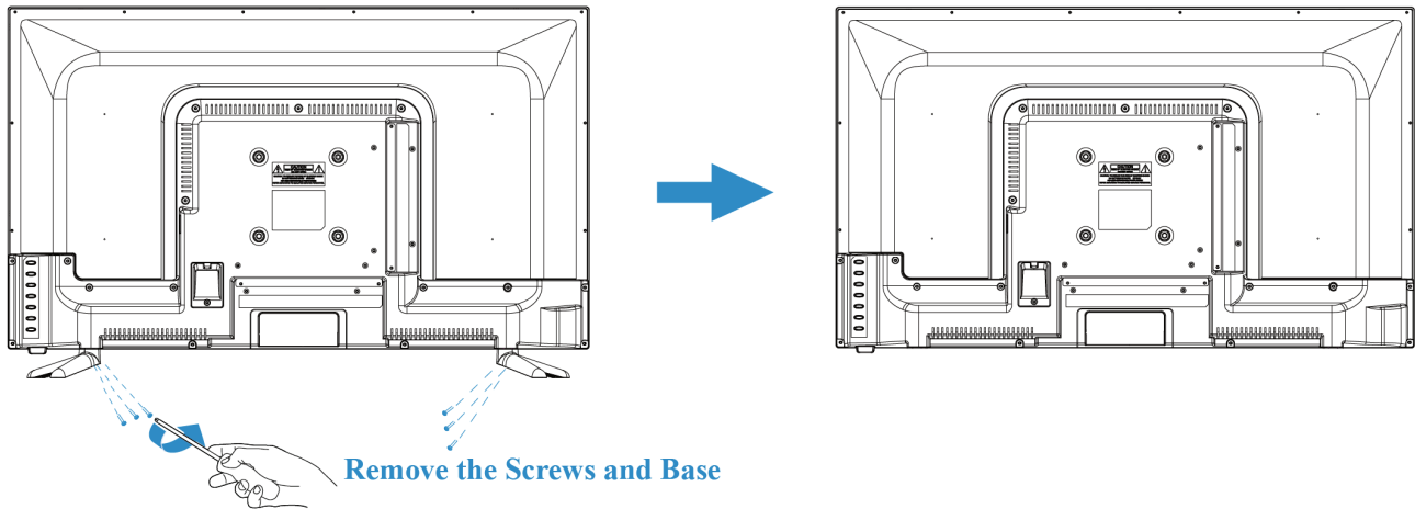
ABBILDUNG 1. INSTALLIEREN UND ENTFERNEN DES STÄNDERS
